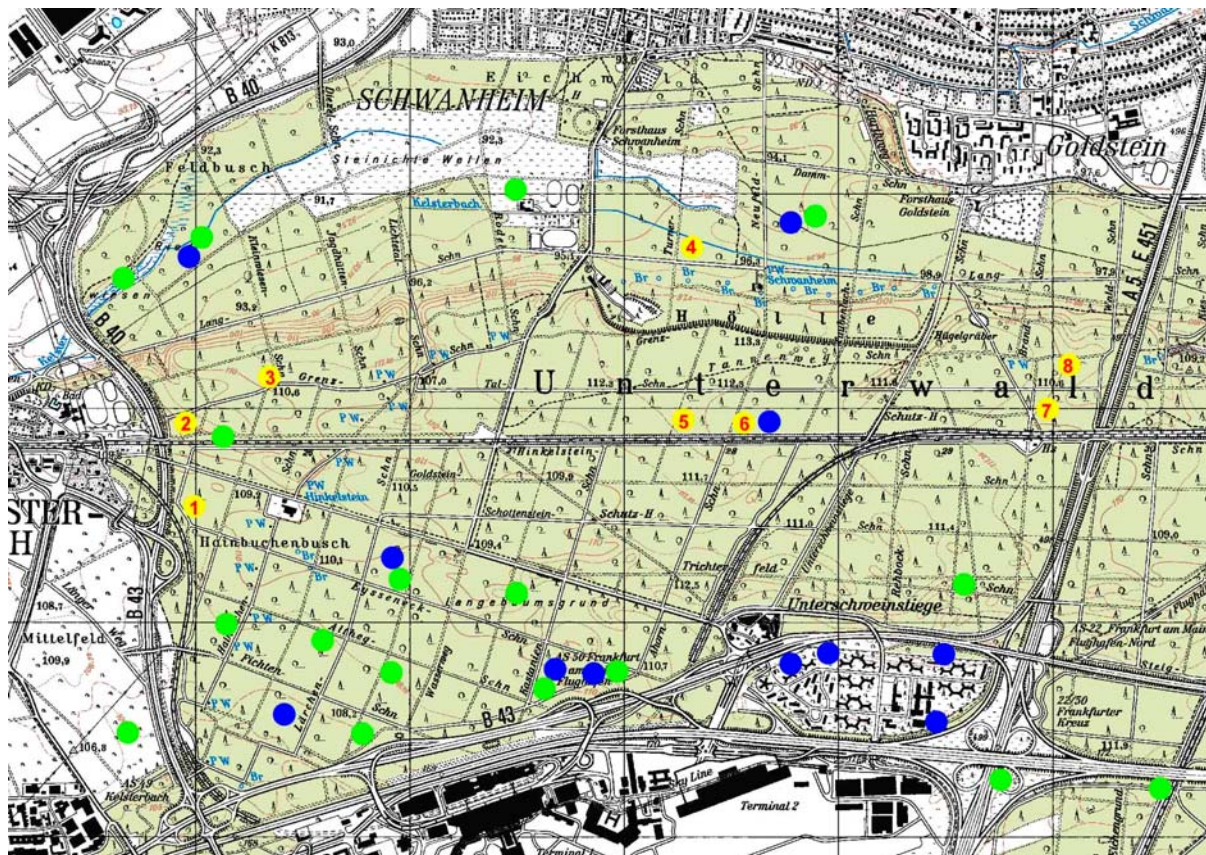
Abb. 7: Verteilung der Probestellen der Vergleichsstandorte im Schwanheimer Wald. (1-8; frühere Untersuchungen: grüne Punkte = Bodenfallenstandorte; blaue Punkte = Stammelektorstandorte) (ohne Maßstab).
